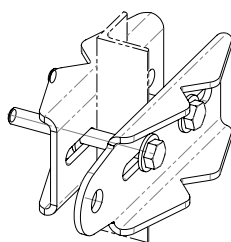
REF : 100479 Extrémité inox réglable (pour tube rond diamètre 60 mm max ou tube carré section 90 mm max).
