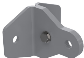
REF : 100153 Extrémité inox pour support béton. Fixation : 2 M12
