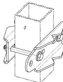
REF : 100479 Extrémité inox réglable (pour tube rond diamètre 60 mm max ou tube carré section 90 mm max).
