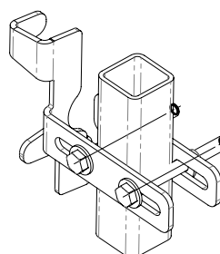
REF : 100480 Intermédiaire inox réglable (pour tube rond diamètre 60 mm max ou tube carré section 90 mm max). A installer tous les 8 mètres.
