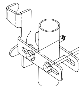
REF : 100480 Intermédiaire inox réglable (pour tube rond diamètre 60 mm max ou tube carré section 90 mm max). A installer tous les 8 mètres.
