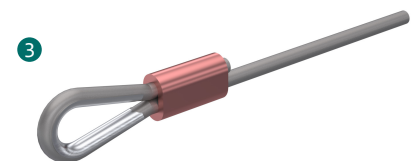
REF : 100478 Ensemble sertissage pour câble inox + cosse coeur inox diamètre 8 mm.
