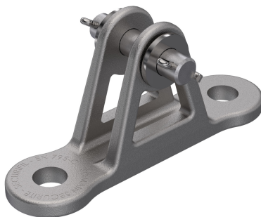
REF : 102422 Extrémité bi-ancrage inox auto. Fixation : 2M12
