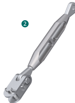
REF : 100122 Tendeur inox oeil/chape, permet le réglage de la tension de la ligne de vie lors de l'installation.
